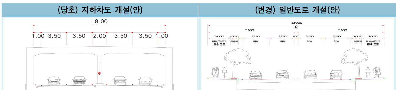
[그림 2] ○○○○지구 지하차도 설계변경 현황
